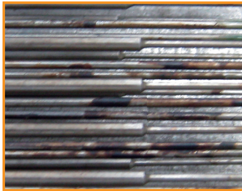
エゼクターピン
